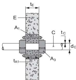
Tubes plastiques avec collier CFS-C
