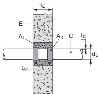
Tubes plastiques avec bande CFS-W
